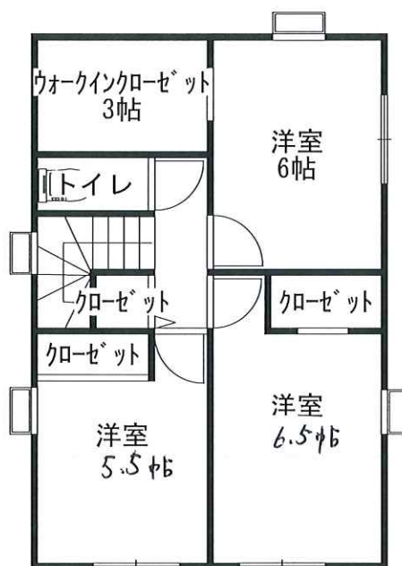
2階平面図
